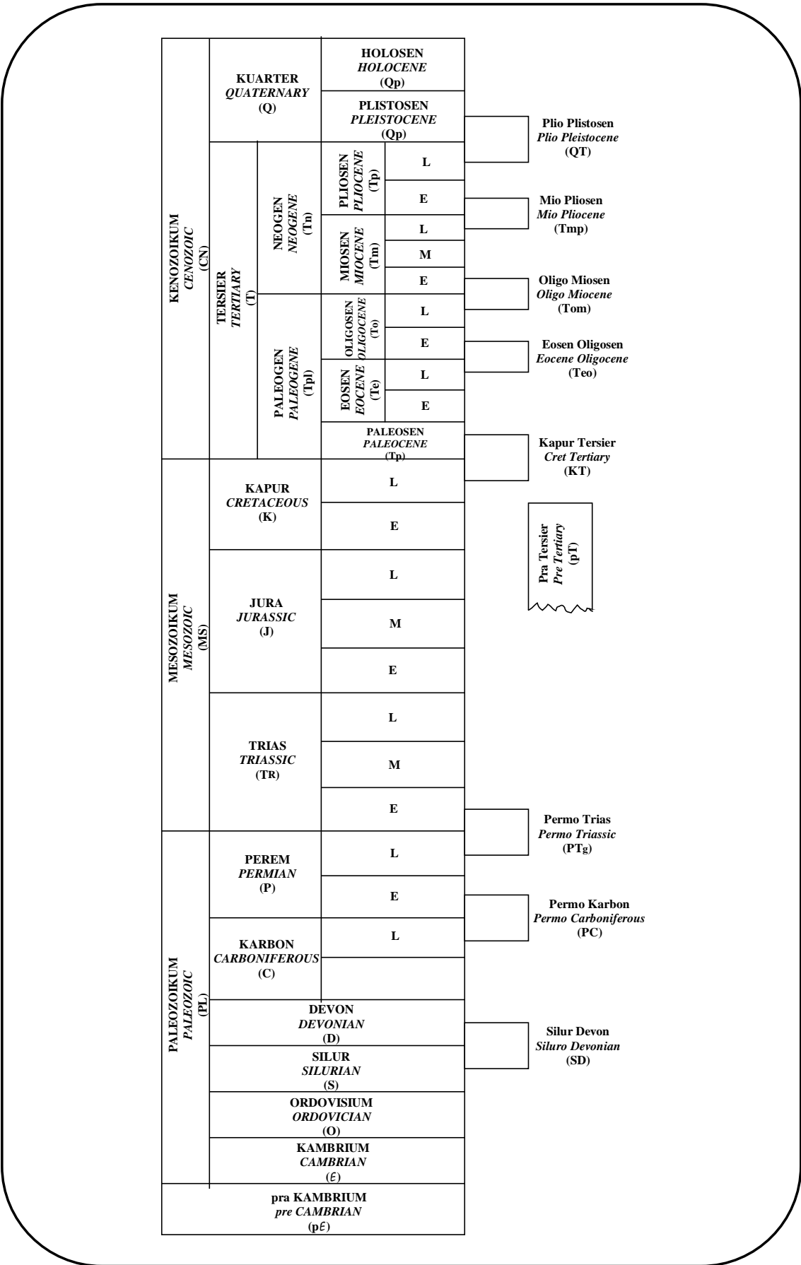
Gambar 1. Singkatan Huruf satuan kronostratigrafi yang digunakan pada peta geologi
