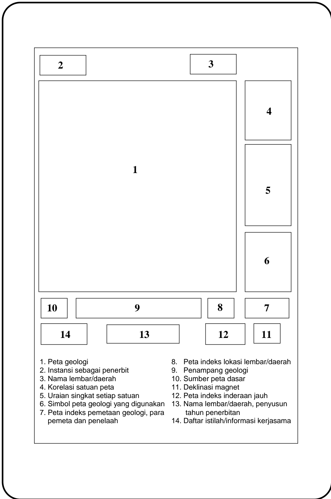
Gambar 7. Tata letak keterangan pinggir pada peta geologi
