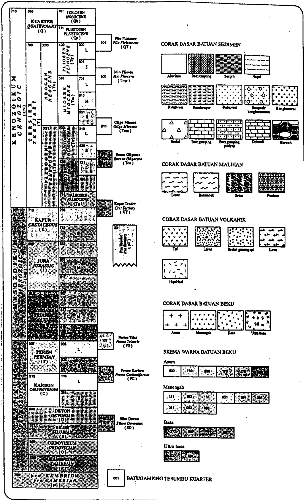
Gambar 3. Skema warna dan corak dasar yang digunakan dalam peta geologi
